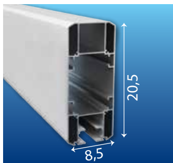
ΟΔΗΓΟΣ PERGO IDEAL 205
